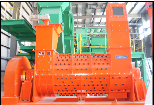
⑧ ラベル剥離機
